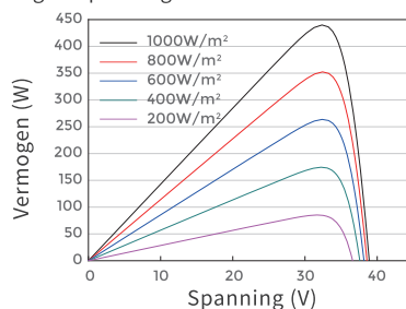
Vermogen-spanningscurve JAM54D41-440/LB
