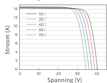
Stroom-spanningscurve JAM54D41-440/LB
