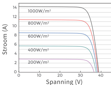
Stroom-spanningscurve JAM54D41-440/LB
